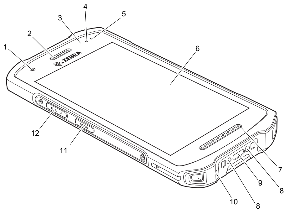
Figura 1 Vista frontal
