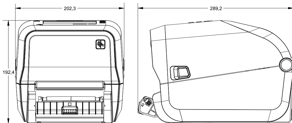
Impressora com distribuidor de etiquetas (aberto)
