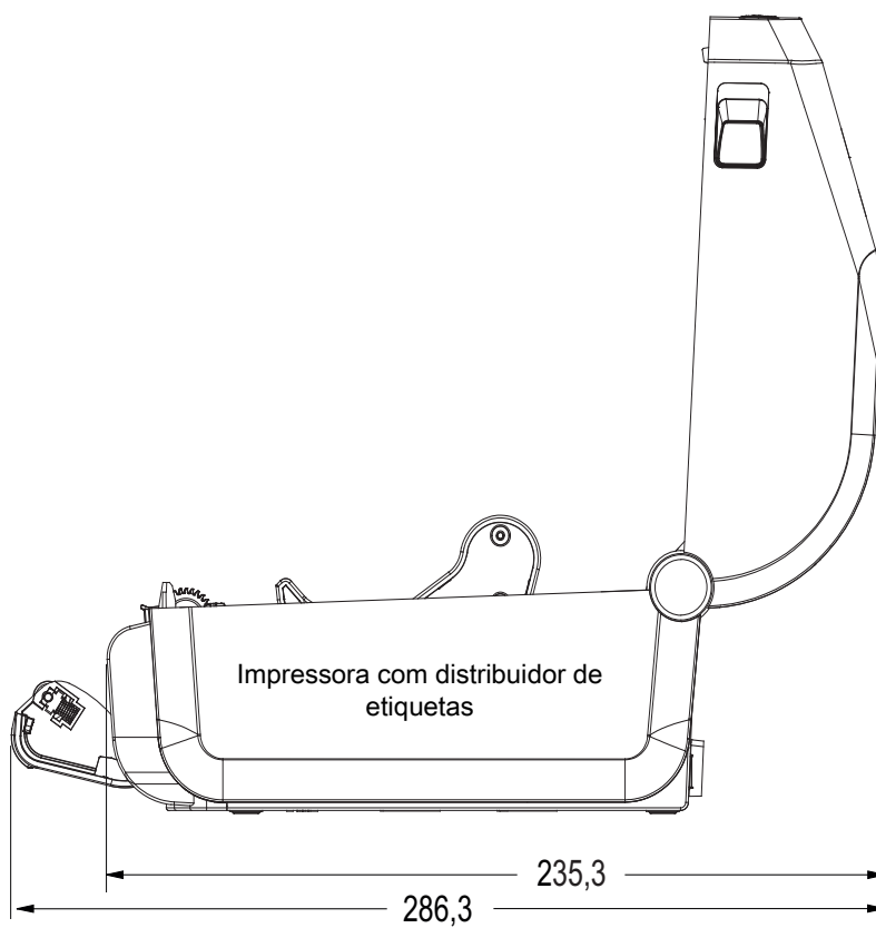
Impressora com distribuidor de etiquetas
