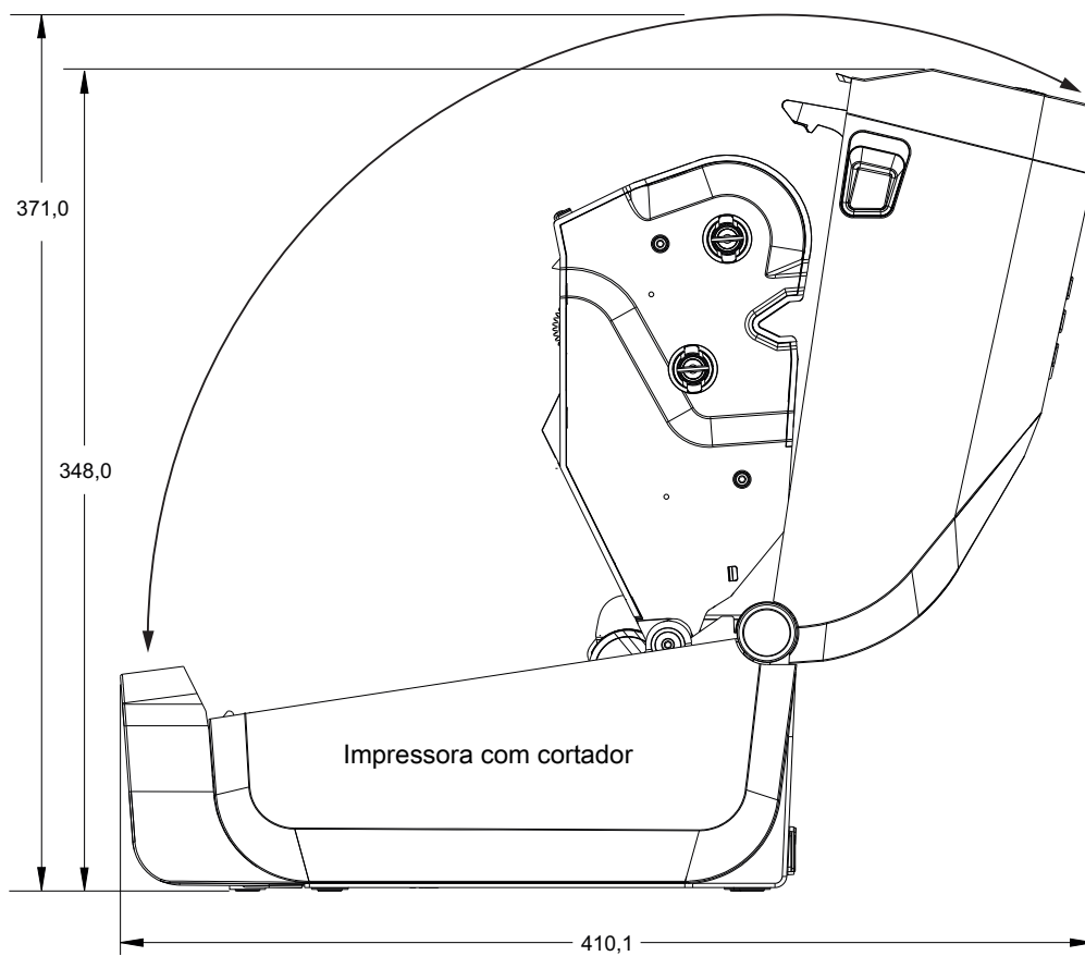
Impressora com cortador
